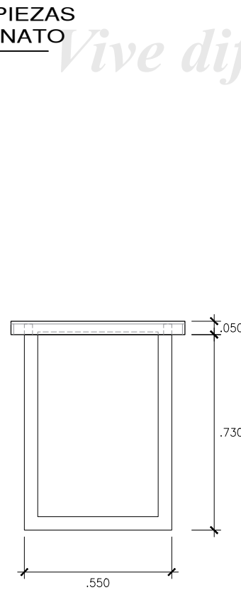
DESPIECE DE PORCELANATO ESCALA 1:25
